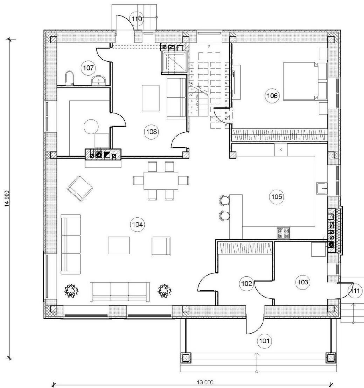
План 1 этажа
