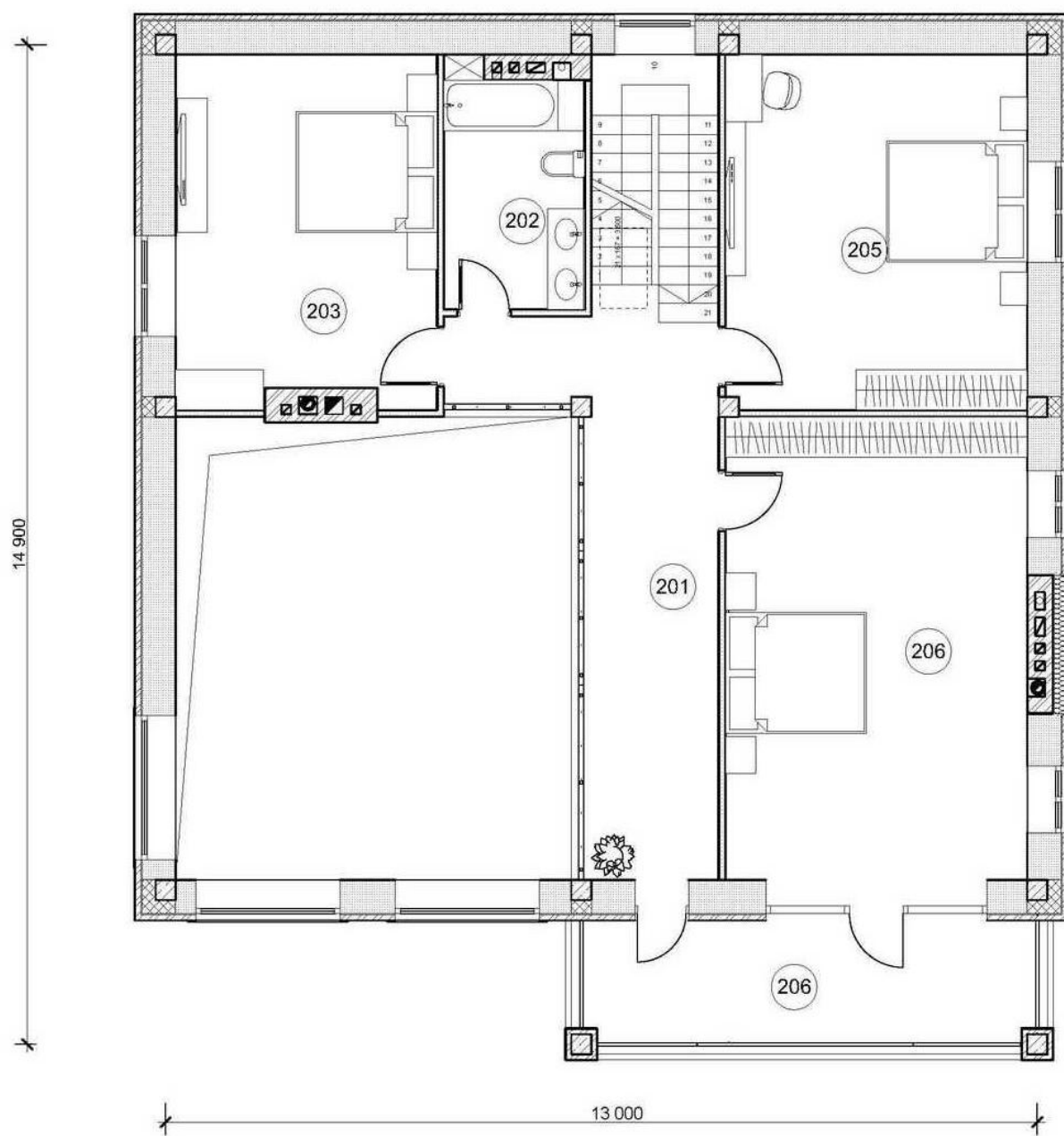
План 2 этажа
